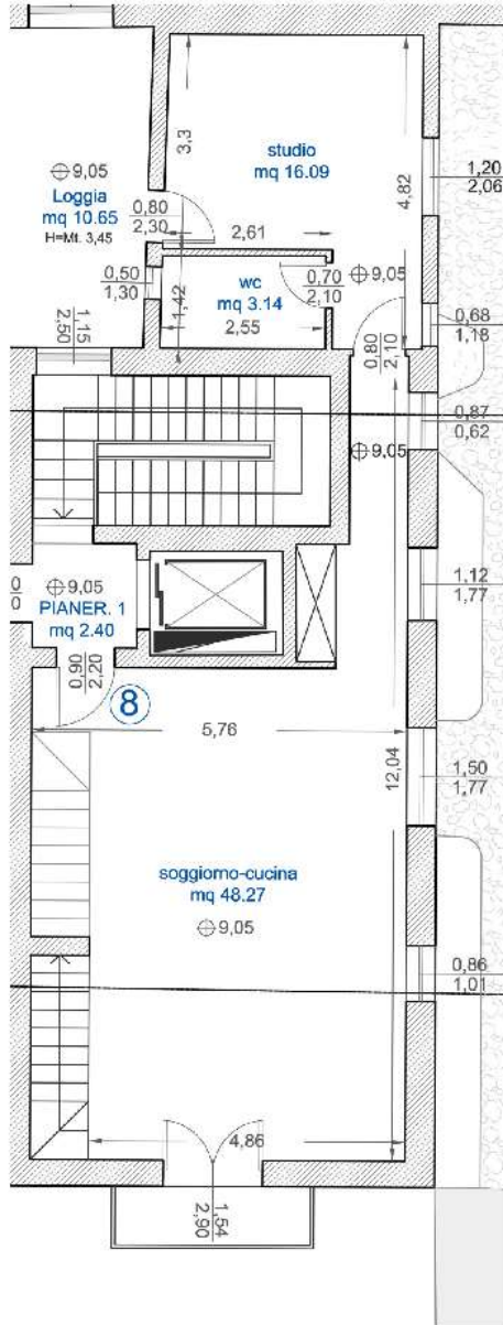
SECONDO PIANO_ZONA GIORNO
