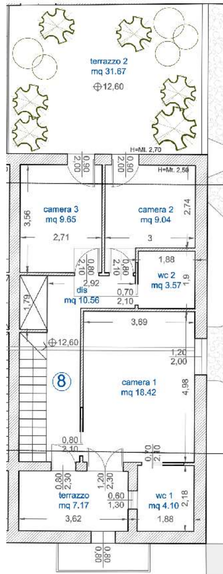
PIANO TERZO_ZONA NOTTE
